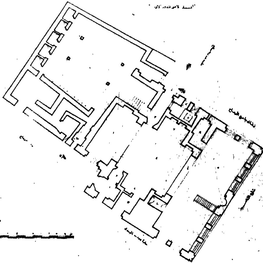
شكل (١٩) يبين مسقط أفقى لمدرسة قانى باى الرماح بجى الناصرية بالسيدة زينب رضوان الله عليها
